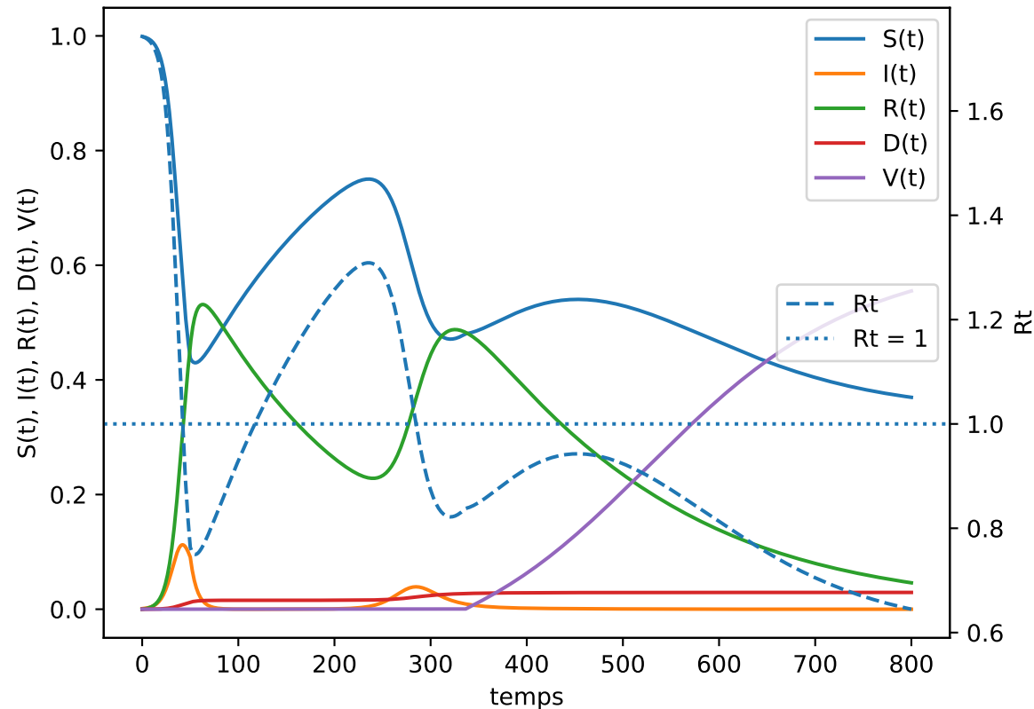
Modélisation covid avec vaccination sigmoïde logistique
